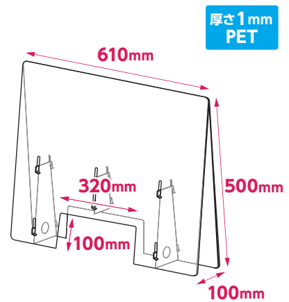
飛沫防止透明 パーテーション窓あきタイプ
