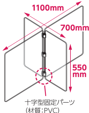
品番 051229 長方形タイプ(1100×700mm)
