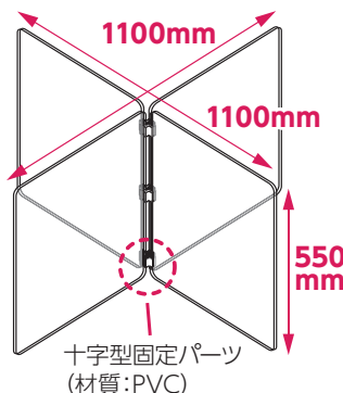
品番 051228 正方形タイプ(1100×1100mm)
