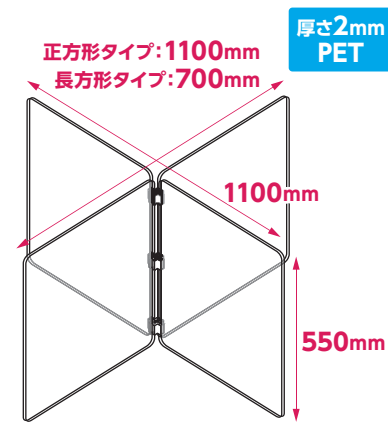
飛沫防止十字型 卓上パーテーション
