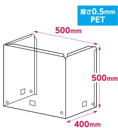
飛沫防止3面ガード
